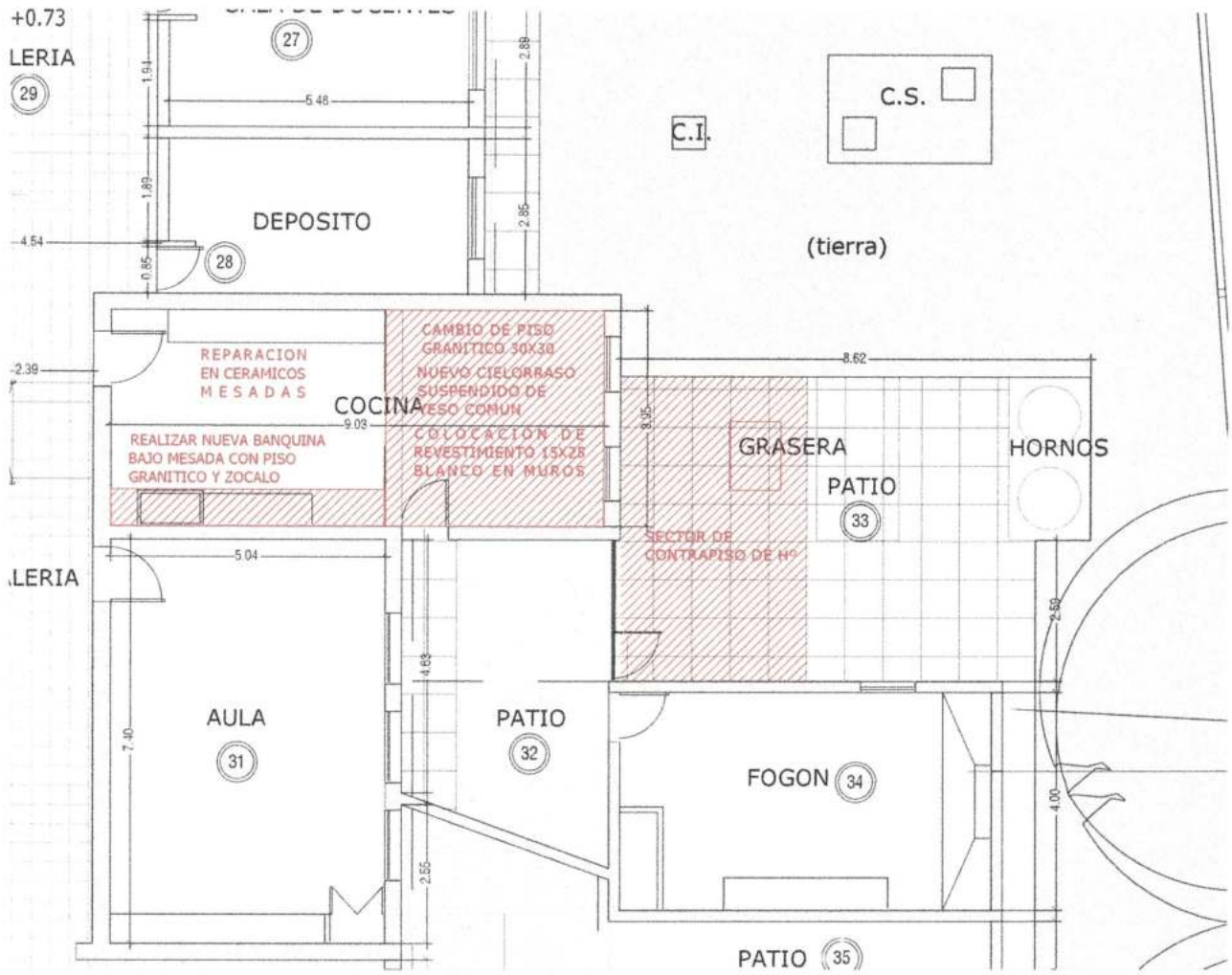
Detalle bajo mesada granito
