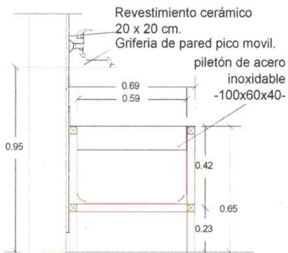
Detalle de Piletón de Acero Inoxidable
